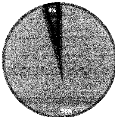
Gráfico 4: Orientação Sexual
